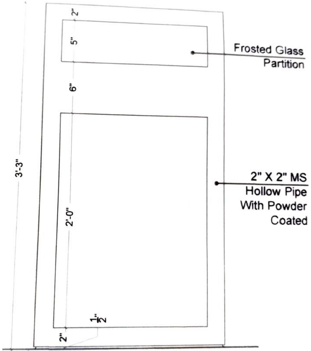
ELEVATION 02
